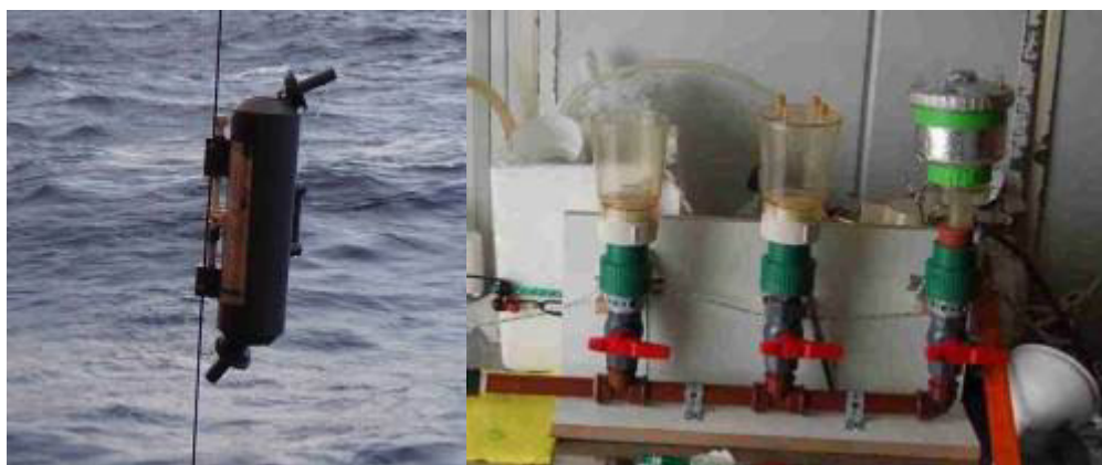
Figura 1. (A) Equipo utilizado en el muestreo de agua botella Niskin 5Lts. (B) Sistema para el filtrado de las muestras de agua (vaso colector de la izquierda).
