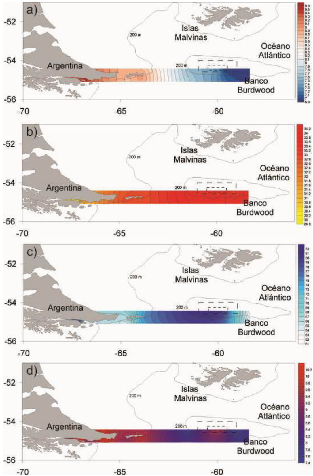
Figura 2. Distribución espacial de a) temperatura (°C), b) salinidad (ups), c) porcentaje de oxígeno disuelto (mg/l) y d) pH registrados a 10 m de profundidad con un multi-parámetro HI9892 Hanna.
