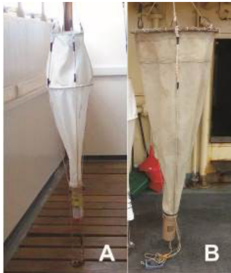
Figura 1. Equipo utilizado en el muestreo de plancton. Red de fitoplancton de 25 \mu\text{m} (A); red de zooplancton de 200 \mu\text{m} (B).
