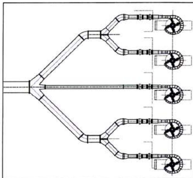
Esquema desde Trifurcación hasta Turbina
