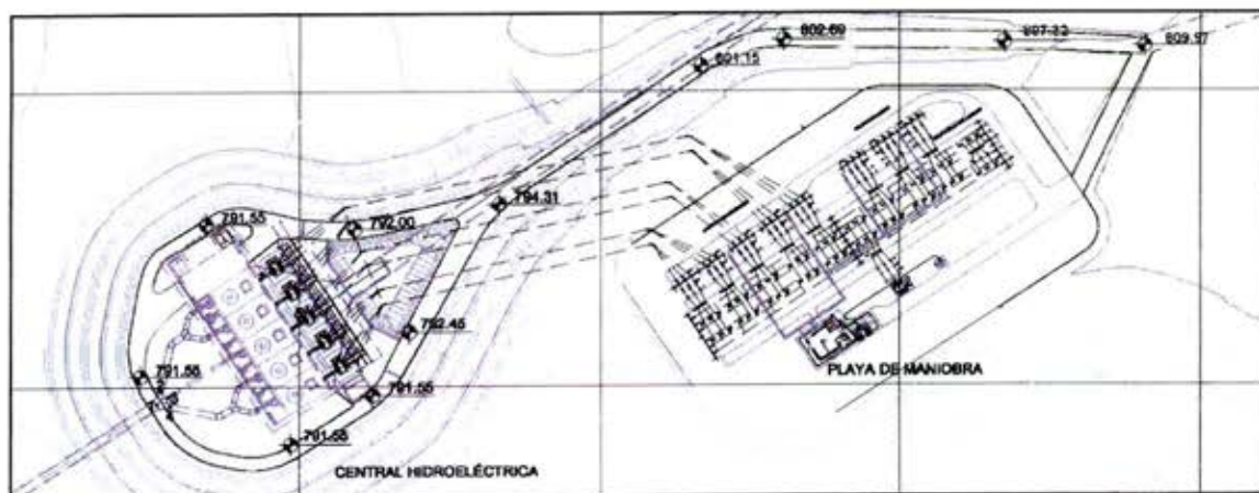
Implantación General de la Central Hidroeléctrica
