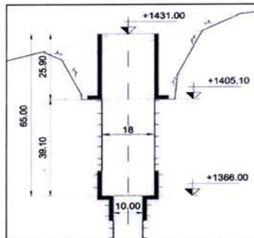
Corta General de Chimenea de Equilibrio
