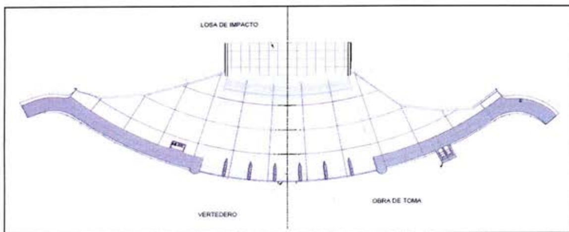
Planta Típica de la Presa
