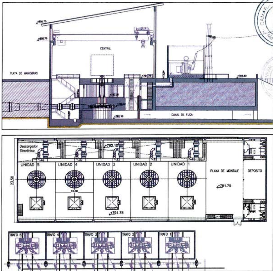
Planta y Corte de Central Hidroeléctrica
