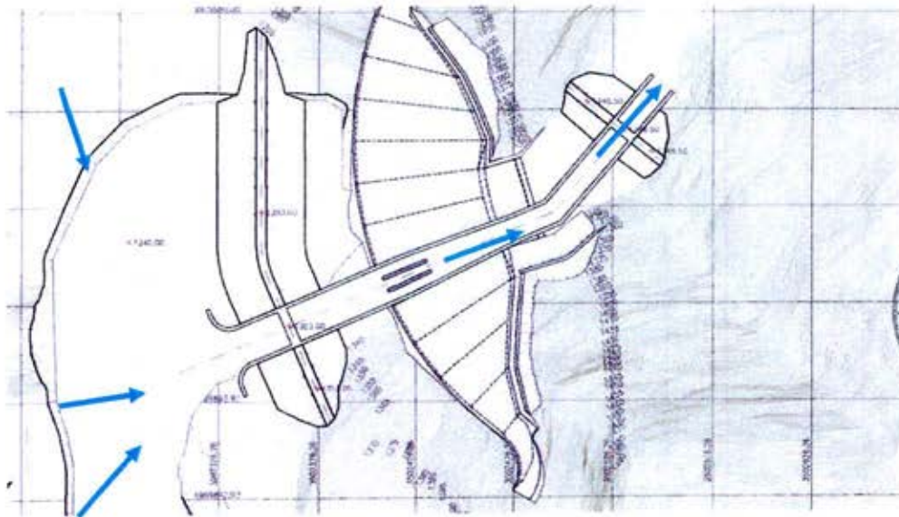
Etap 3 de Desvío del Río - Remoción de Ataguías Provisorias de 1ra etapa y Construcción de Ataguías de Desvío del Río
