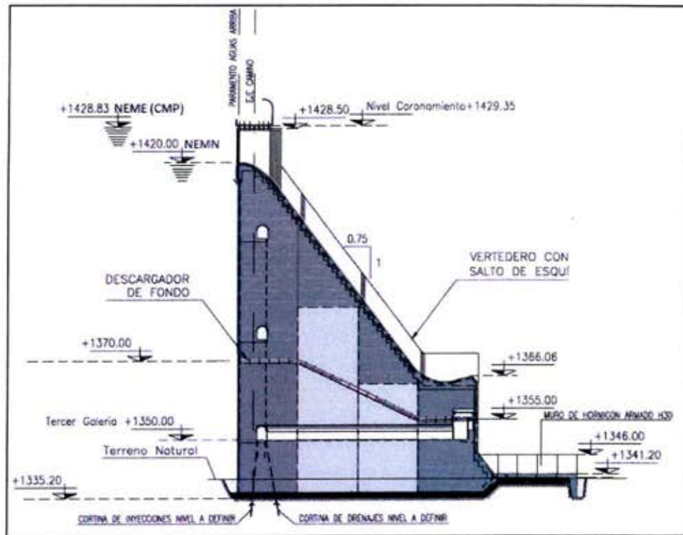
Perfil Tipo de la Presa de Hormigón
